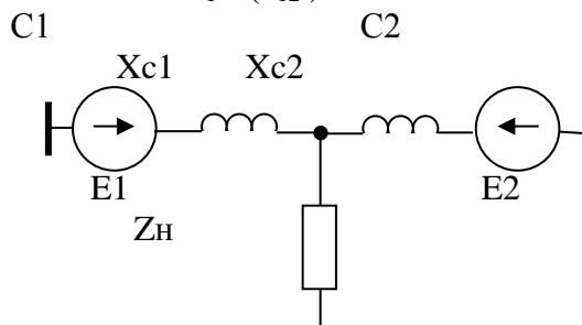
Рис. 3 Схема замещения электропередачи для расчета действительного предела мощности при нагрузке Z_H , заданной постоянным сопротивлением
