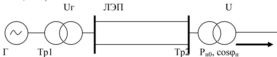
Рис. 1 Схема электропередачи
